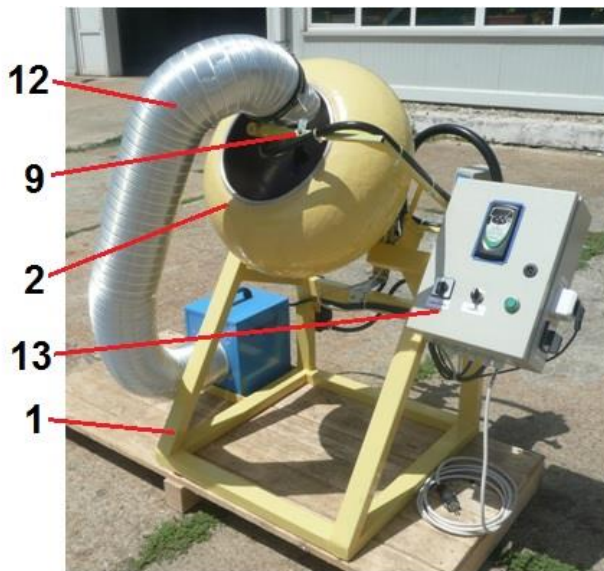
Masina de tratat seminte ETS-INMA
